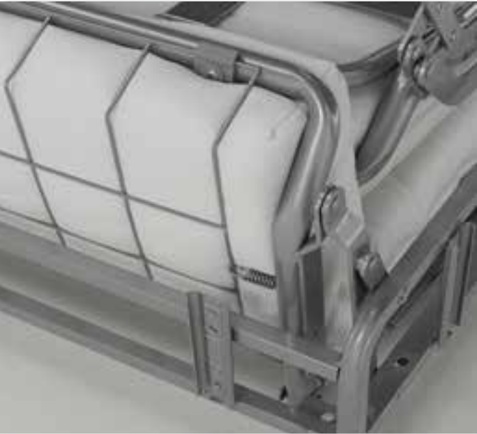
Szczegół zamykania mechanizmu Grecale de Luxe
